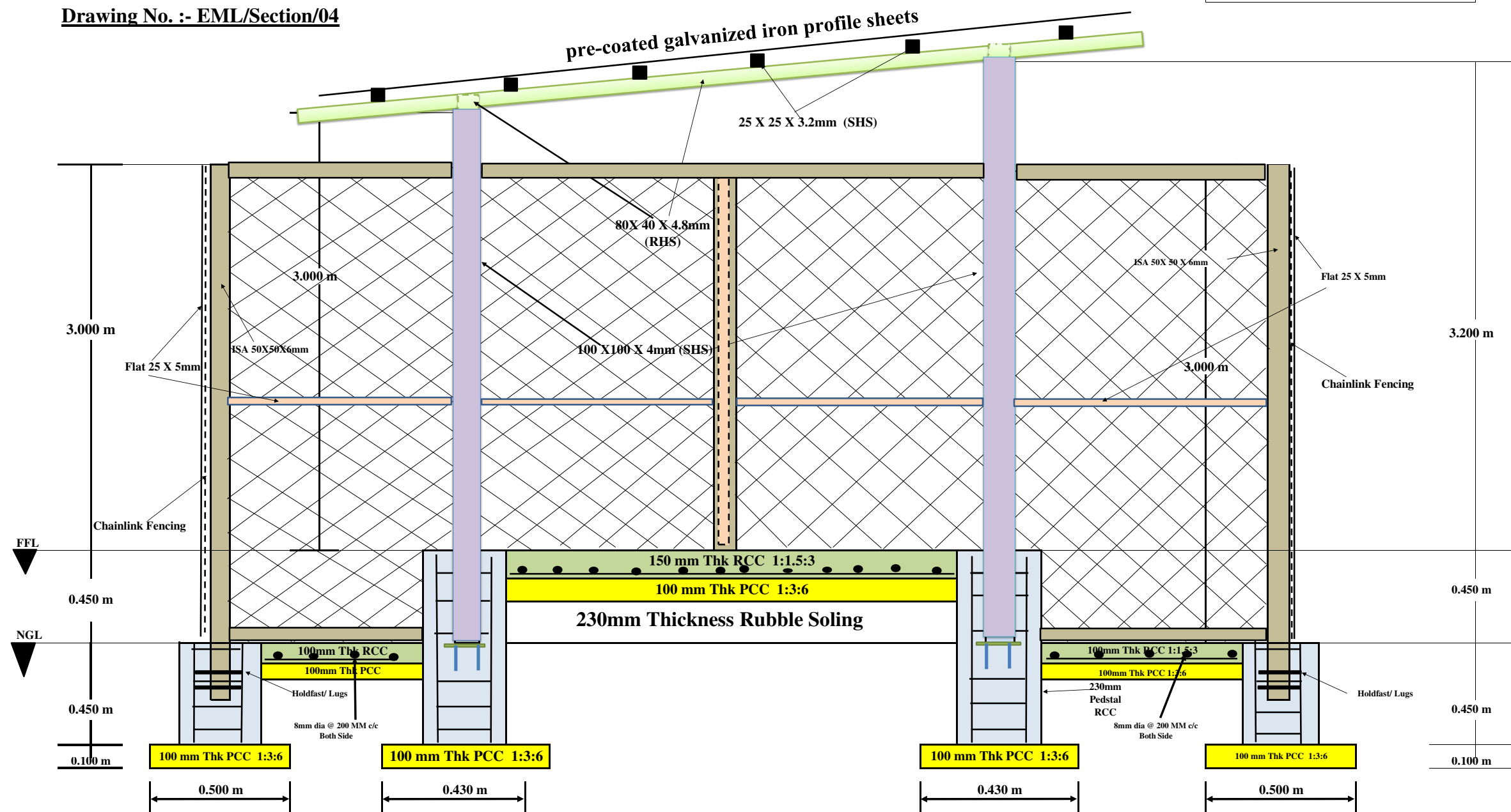
Section D-D
