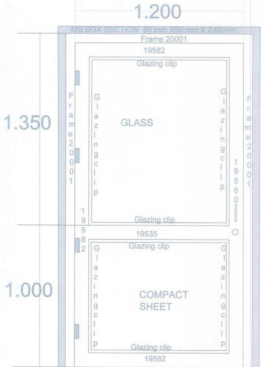
TYP. DETAILS OF DOOR
